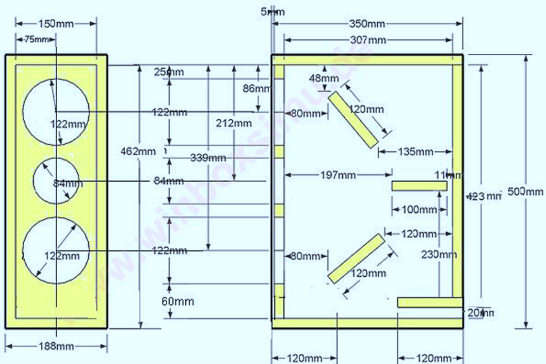
not0815 - Selbstbau-Lautsprecher - www.winboxsimu.de Bauplan Modell: BlueFlex - © Sven Patelscheck 2009
